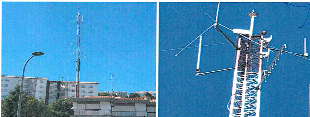
Figura 1 – Equipamentos Rádio na torre do CDOS da Guarda para ligação à TAR de Jarmelo, Vilar Formoso e São Cornélio.
